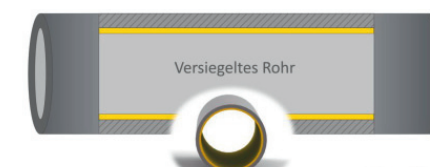
... zu schliessen, werden die Heizungsrohre durch ein Versiegelungsverfahren von innen versiegelt.
